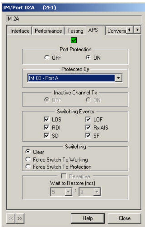
Figure 5 – Dual E1 IM Configuration Dialog APS Tab
