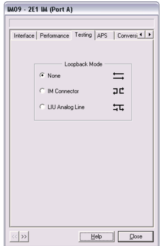
Figure 4 – Dual E1 IM Configuration Dialog Testing Tab
