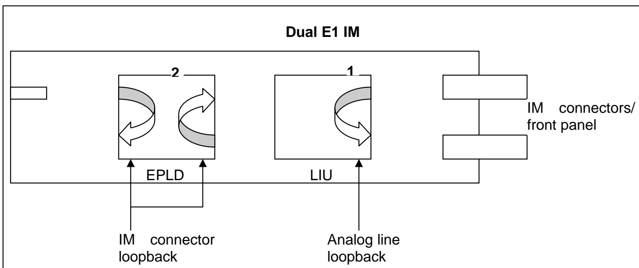
Figure 7 – E1 IM loopback options
